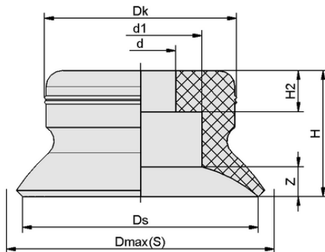
设计数据 PFG 20 FPM-65 N006
