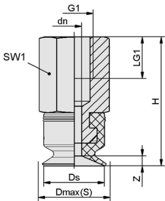
设计参数 PFYN 10 PU-55 M5-IG
