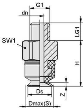
设计参数 PFYN 10 SI-55 M5-AG
