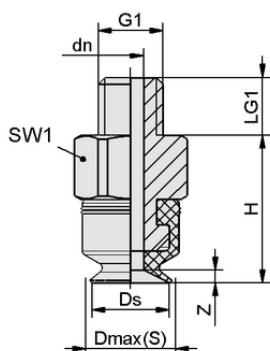
设计参数 PFYN 3.5 FPM-65 M3-AG
