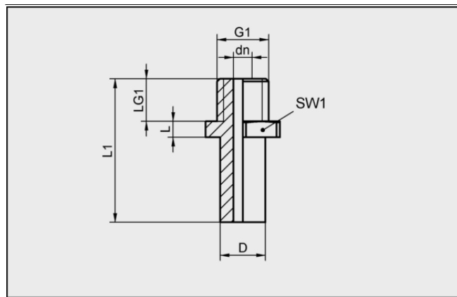
设计参数 SA-NIP N002 M3-AG DN70
