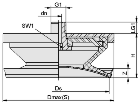
设计参数 SPL-HT 90 FPM-F-65 G1/4-AG
