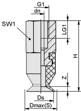
设计参数 SGAN 16 SI-55 G1/8-IG
