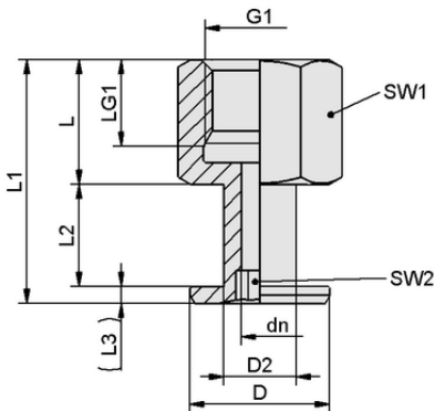
设计参数 SA-NIP N008 G1/8-IG DN350
