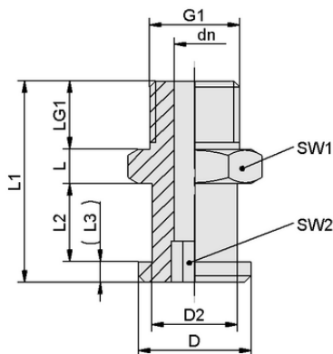
设计数据 SA-NIP N006 G1/8-AG DN200
