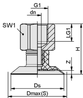
设计参数 SGPN 15 NK-40 G1/8-IG
