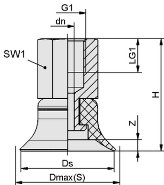
设计参数 PFYN 40 NBR-CO-55 G1/8-IG
