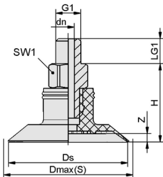
设计参数 SGPN 34 NK-40 G1/4-AG
