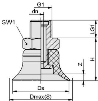
设计参数 PFYN 40 HT1-60 G1/8-AG
