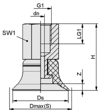
设计参数 PFYN 50 HT1-60 G1/8-IG
