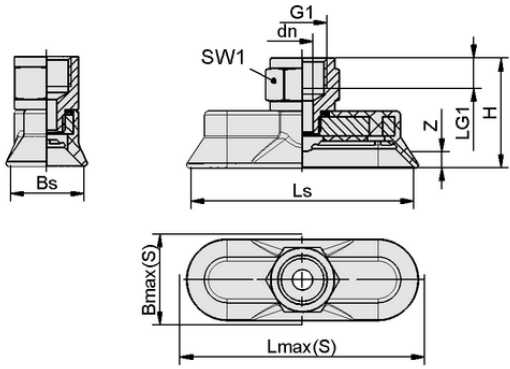
设计参数 SAOG 95x40 NBR-45 G3/8-IG
