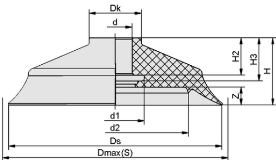
设计参数 SHF 50 NK-45 N041 MOS
