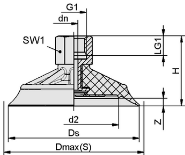
设计数据 SHFN 70 NK-45 G1/4-IG MOS
