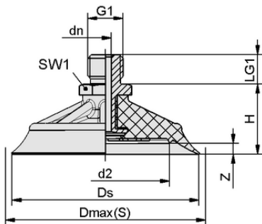
设计参数 SHFN 70 NK-45 G1/4-AG TV
