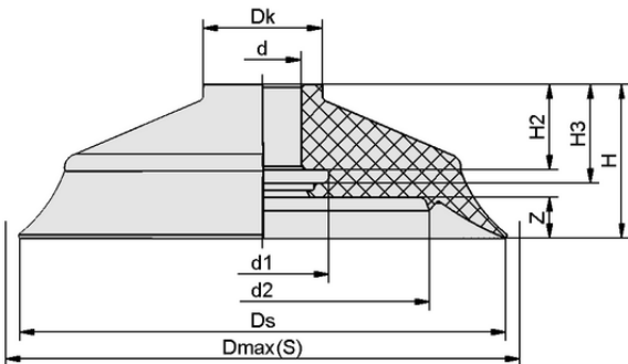
设计参数 SHF 85 NK-45 N041
