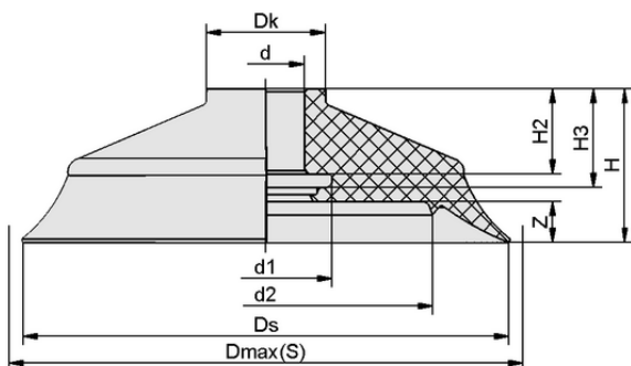
设计参数 SHF 85 NK-45 N041 MOS
