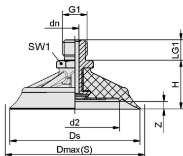
设计参数 SHFN 85 NK-45 G1/4-AG TV
