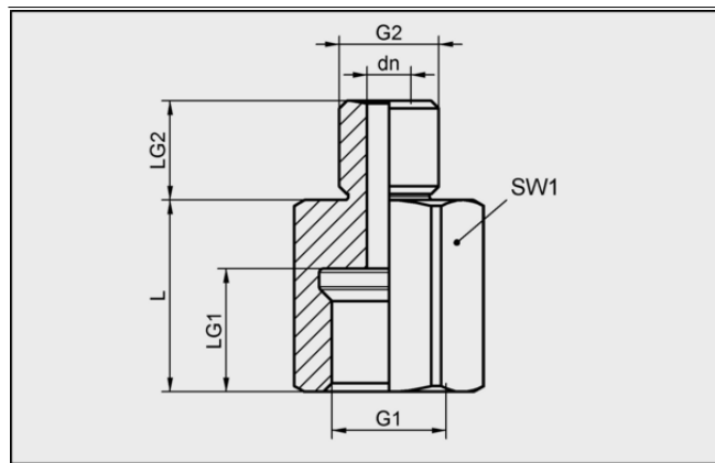
设计数据 SA-NIP N009 G1/4-IG DN440
