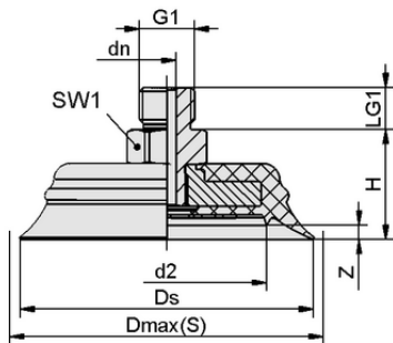
设计参数 SHFN 70 NK-45 G1/4-AG E
