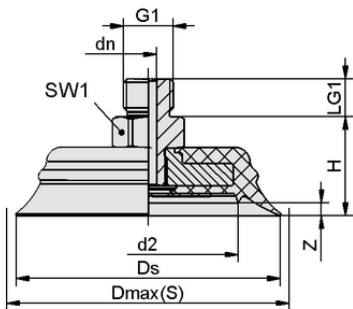
设计参数 SHFN 70 NK-45 G1/4-AG E MOS
