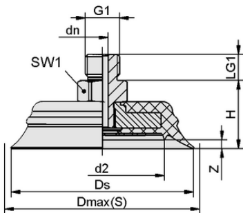
设计参数 SHFN 70 NK-45 G1/4-AG E TV
