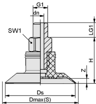
设计数据 SGPN 15 HT1-60 M5-AG
