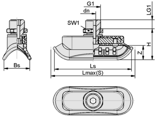
设计参数 SAOK 70x25 HT2-65 G1/4-AG
