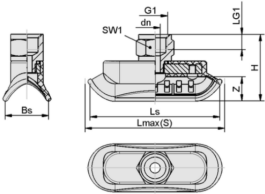
设计参数 SAOK 70x25 HT2-65 G3/8-IG
