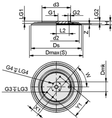
SGF 400 EPDM-55 G1/2-IG
