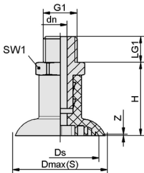
设计参数 SGPN 35 SI-50 G1/4-AG
