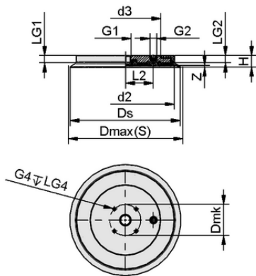
设计数据 SGF 125 HT1-60 G1/4-IG
