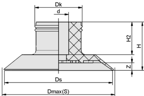
设计参数 SGP 34 FPM-65 N033
