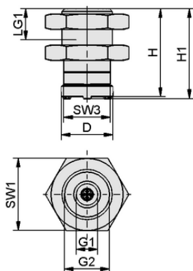
设计参数 SBS 10 SF M5-IG AL
