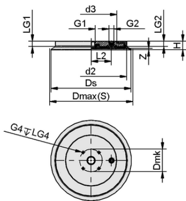
设计参数 SGF 125 HT1-60 G3/8-IG
