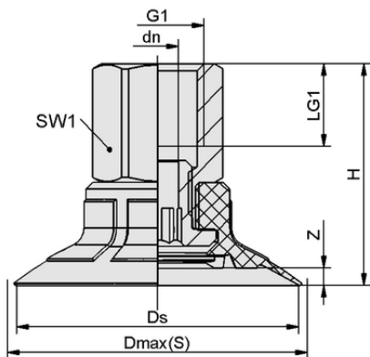
设计数据 SPF 50 ED-65 G1/4-IG
