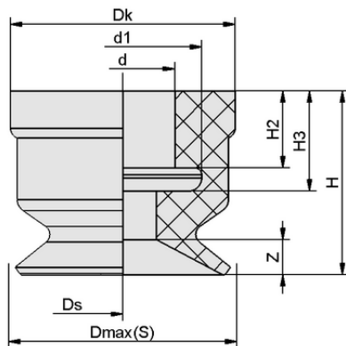
设计参数 SUF 8 HT1-60 SC020
