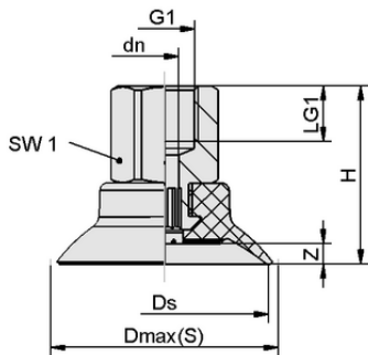
设计参数 SUF 30 SI-55 G1/8-IG
