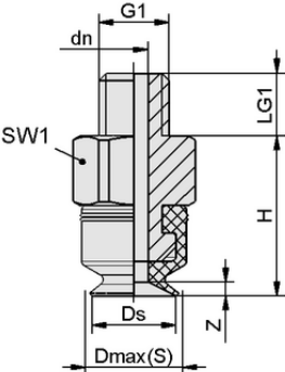
设计参数 PFYN 8 NBR-ESD-55 M5-AG
