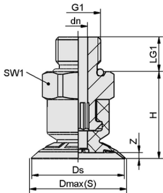
设计数据 SFF 20 SI-55 G1/8-AG
