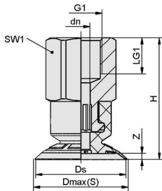
设计参数 SFF 25 EPDM-45 G1/8-IG
