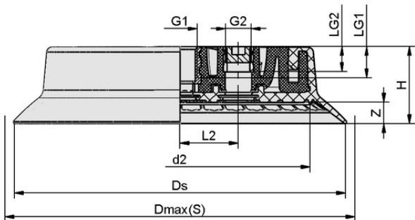
设计参数 SUF 125 NBR-60 G1/4-IG VRS
