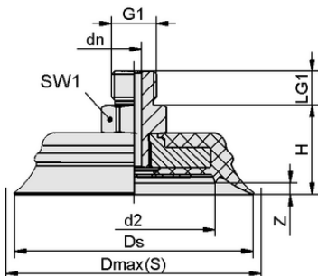
设计参数 SHFN 50 NK-45 G1/4-AG E
