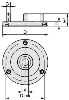
设计参数 SBS 20 SF TH M1.6-AG AL
