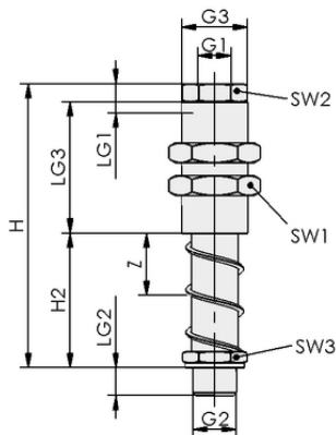
Design data FSTE G1/8-AG 15 VG
