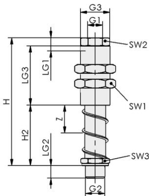
Design data FSTE-HD G1/2-AG 25
