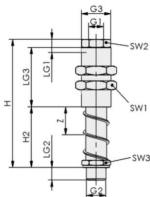
设计参数 FSTE-HD G1/2-AG 90
