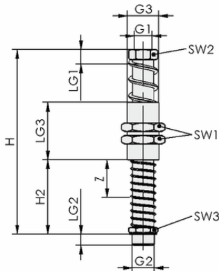
设计参数 FSTA-HD G1/2-AG 25
