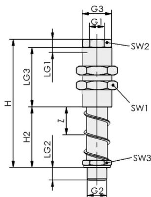
Design data FSTE-HD G3/8-AG 75 VG
