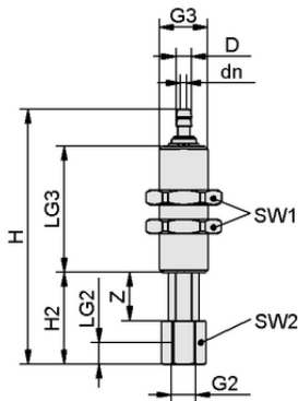
设计参数 FSTIm M5-IG 6/4 A 10 VG-IN
