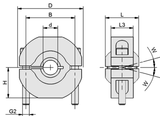
Design data HTR-UNI 2N FSTI
